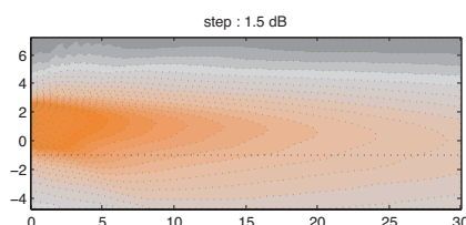
Step Array SA300S+ directivité verticale : niveau sonore pour les octaves de la parole (500Hz-1kHz-2kHz) dans le plan vertical médian.
