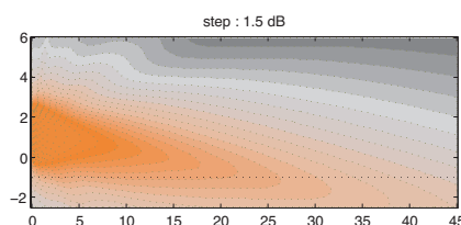
Step Array SA300P+ directivité verticale : niveau sonore pour les octaves de la parole (500Hz-1kHz-2kHz) dans le plan vertical médian.
