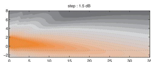
Step Array SA230P+ directivité verticale : niveau sonore pour les octaves de la parole (500Hz-1kHz-2kHz) dans le plan vertical médian.
