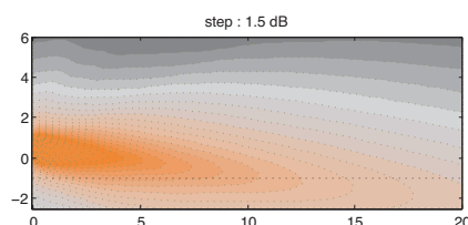
Step Array SA150P+ directivité verticale : niveau sonore pour les octaves de la parole (500Hz-1kHz-2kHz) dans le plan vertical médian.
