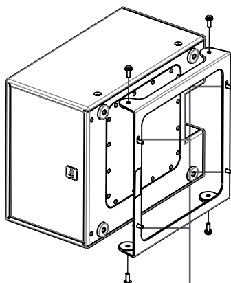
Trous de fixation pour une installation sur un pan de mur adapté.
