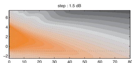
Step Array SA400P directivité verticale : niveau sonore pour les octaves de la parole (500Hz-1kHz-2kHz) dans le plan vertical médian.
