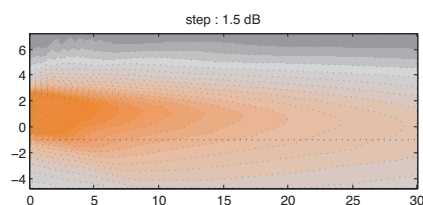
Step Array SA250S directivité verticale : niveau sonore pour les octaves de la parole (500Hz-1kHz-2kHz) dans le plan vertical médian.
