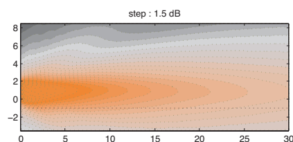
Step Array SA180S directivité verticale : niveau sonore pour les octaves de la parole (500Hz-1kHz-2kHz) dans le plan vertical médian.
