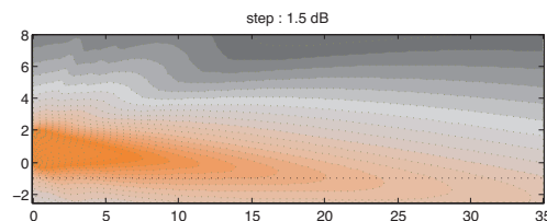
Step Array SA180P directivité verticale : niveau sonore pour les octaves de la parole (500Hz-1kHz-2kHz) dans le plan vertical médian.
