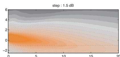
Step Array SA100P directivité verticale : niveau sonore pour les octaves de la parole (500Hz-1kHz-2kHz) dans le plan vertical médian.
